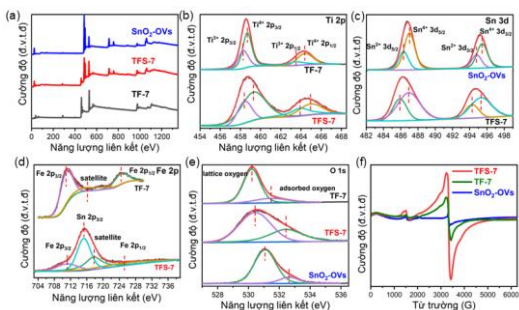
Hình 5.4. Phổ XPS tổng quát (a) và phổ phân giải cao của Ti 2p (b), Sn 3d (c), Fe 2p (d), O 1s, phổ EPR (f) của TF-7, SnO 2 -OVs và TFS-7.
