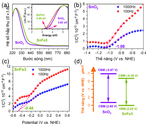
Hình 4.10. (a) Phổ UV-vis DRS của \text{SnO}_2 và \text{SnFe}_3 (hình nhỏ kèm theo biểu đồ Tauc tương ứng, biểu diễn (\text{ah}\nu)^2 với năng lượng (h\nu) ); (b) Biểu đồ Mott-Schottky của \text{SnO}_2 ; (c) Biểu đồ Mott-Schottky của \text{SnFe}_3 ; and (d) cấu trúc vùng của \text{SnO}_2 và \text{SnFe}_3 .
