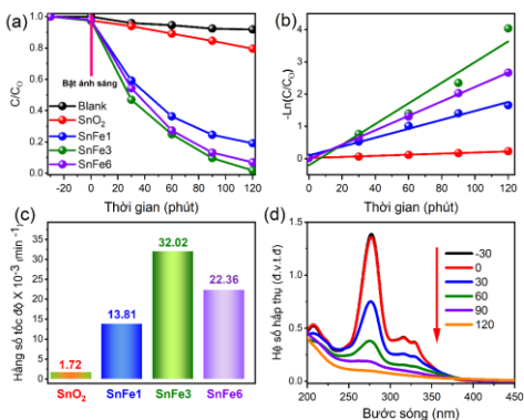
Hình 4.12. Hiệu quả phân hủy quang xúc tác CIP dưới sự chiếu xạ của ánh sáng khả kiến của hệ mẫu \text{SnO}_2:\text{Fe}^{3+} ; đồ thị -\ln(C/C_0) phụ thuộc theo thời gian (b); hằng số tốc độ k của các mẫu \text{SnO}_2:\text{Fe}^{3+} ; phổ hấp thụ UV-Vis của dung dịch CIP trong quá trình phân hủy đối với chất xúc tác SnFe3.
