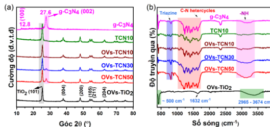
Hình 5.12: (a) Các mẫu nhiễu xạ XRD của \text{g-C}_3\text{N}_4 , \text{OVs-TiO}_2 và các dị thể ( \text{TCN10} , \text{OVs-TCN10} , \text{OVs-TCN30} và \text{OVs-TCN50} ).
