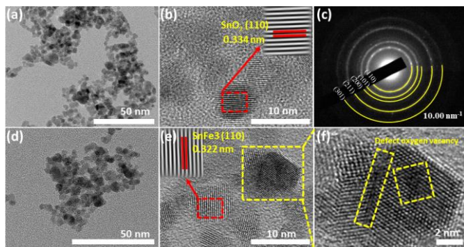
Hình 4.6. Ảnh TEM (a), Ảnh HRTEM (b) và ảnh SAED (c) của mẫu SnO 2 ; Ảnh TEM (d), ảnh HRTEM (e) và phóng to ảnh HRTEM (f) của mẫu SnFe 3 .
