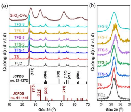
Hình 5.1. (a) Giản đồ nhiễu xạ tia X của TiO 2 ; SnO 2 -OVs và TFS-X; (b) phóng to đỉnh nhiễu xạ (101) của TiO 2 và các mẫu TFS-X.
