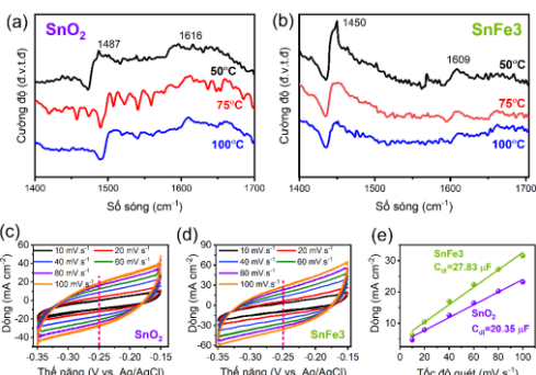
Hình 4.15. Phổ Py-FTIR của (a) \text{SnO}_2 và (b) SnFe3; các chu trình CV ở các tốc độ quét khác nhau của (c) \text{SnO}_2 ; và (d) SnFe3; (e) đồ thị tuyến tính dòng điện phụ thuộc vào tốc độ quét đối với các mẫu \text{SnO}_2 và SnFe3.
