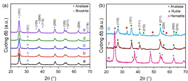
Hình 3.9. Giảm đồ nhiễu xạ tia X của các mẫu TiO 2 pha tạp chất Fe 3+ với các nồng độ: (a)- 0 %mol, (b)- 1 %mol, (c)- 4 %mol, (d)- 8 %mol, (e)- 10 %mol, (f)- 16 %mol and (g)- 25 %mol
