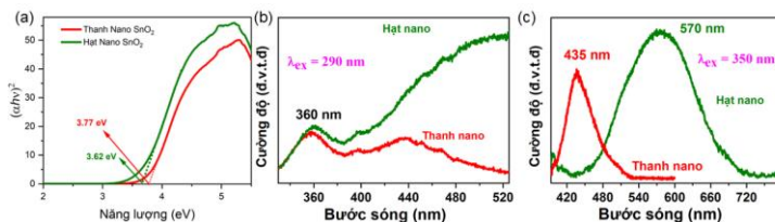
Hình 4.3. Đồ thị (ahv)^2 theo năng lượng photon (a), phổ huỳnh quang kích thích tại bước sóng 290 nm (b) và 350 nm (c) của các thanh và các hạt nano \text{SnO}_2 .
