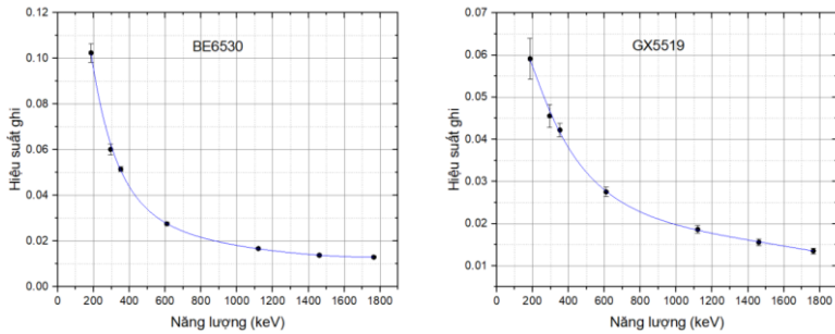
Hình 3.1. Đường cong hiệu suất ghi đối với mẫu đất trên hệ phổ kế gamma BE6530 và GX5519.
