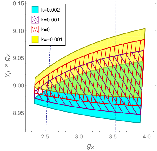
Hình 2.14: Vùng tham số được phép trên mặt phẳng (g_X, y_\mu g_X) cho trường hợp m_{Z'} = 300 GeV, \tau = 1.78 , \delta = 1 và các giá trị khác nhau của k . Các đường chấm gạch và đường đứt nét lần lượt ứng với giới hạn nhiễu loạn của y_\mu và g_X .
