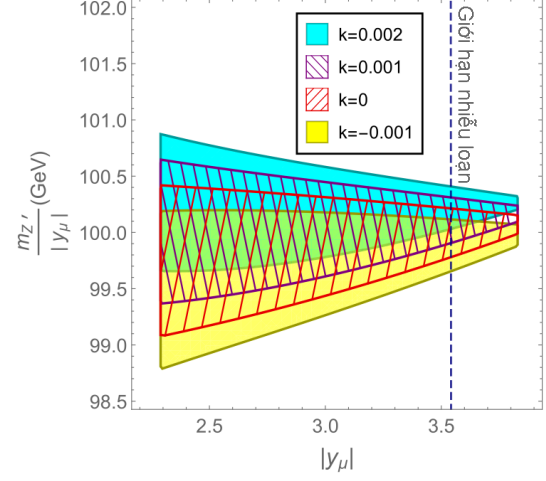
Hình 2.22: Vùng tham số được phép trên mặt phẳng (y_\mu, \frac{m_{Z'}}{|y_\mu|}) cho trường hợp g_X = 3 , \tau = 1.78 , \delta = 1 và các giá trị khác nhau của k .
