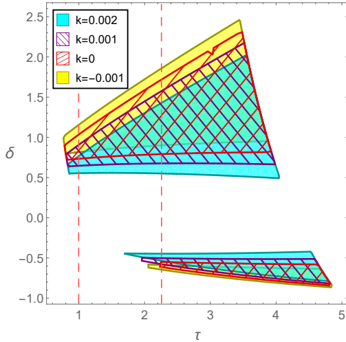
Hình 2.11: Vùng tham số được phép trên mặt phẳng (\tau, \delta) cho trường hợp m_{Z'} = 300 GeV, y_\mu = 3 , g_X = 3 và các giá trị khác nhau của k . Vùng nằm giữa hai đường đứt nét màu đỏ thỏa mãn điều kiện (2.85).
